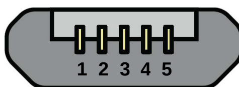
Рис. 2.5 Разъем Micro-USB
