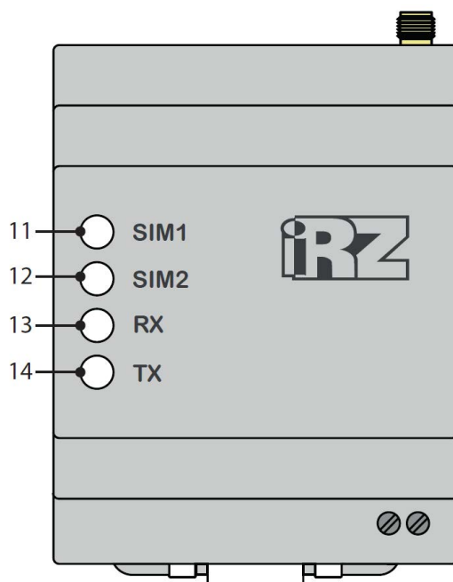
Рис. 2.4 Вид сверху
