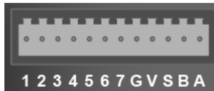
Рис. 3.6. Интерфейсный разъём
