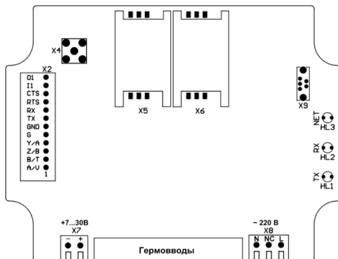
Рис. 16. Разъемы терминалов герметичного исполнения.
