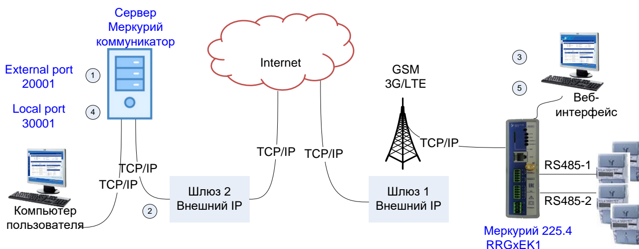
Рисунок 2.1 – Схема работы в режиме «прозрачного канала»
