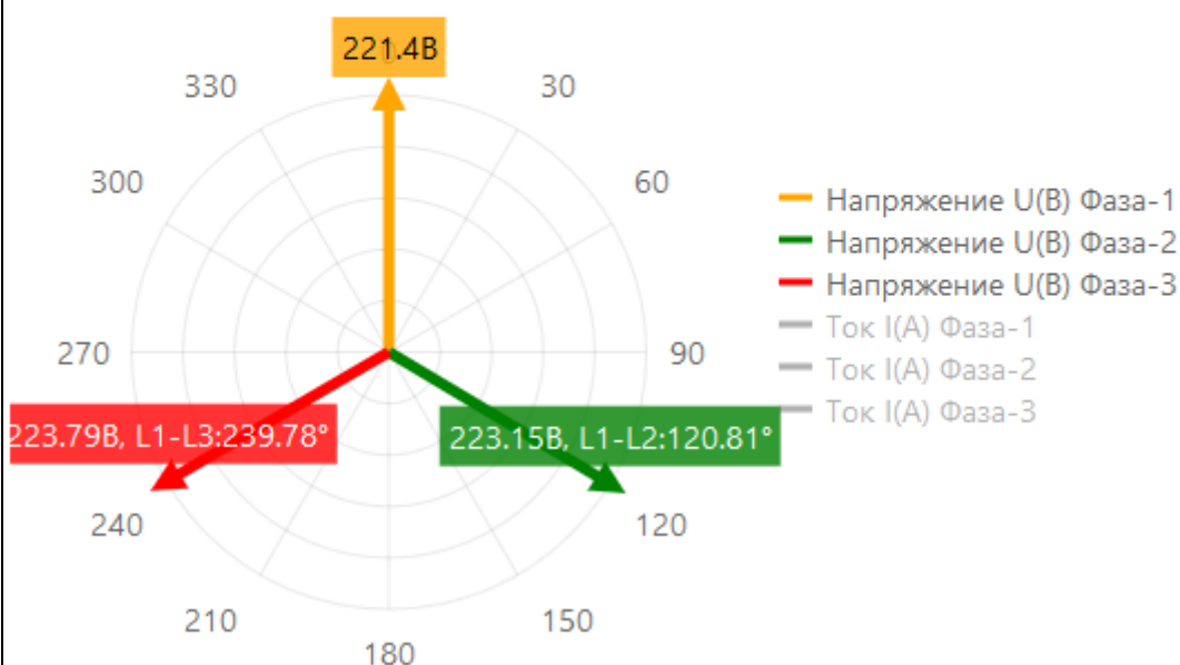
Пофазная векторная диаграмма
