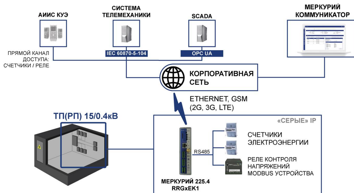
Рисунок 1.3 – Архитектура системы
