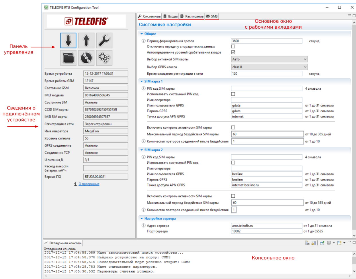
Рис. 42. RTU Configuration Tool. Стартовый вид.
