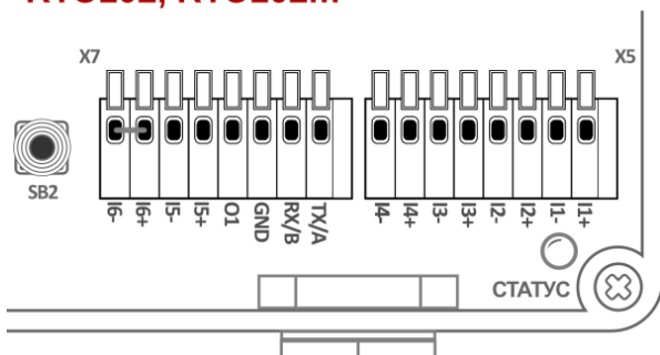
Рис. 6. Контакты клеммных блоков.
