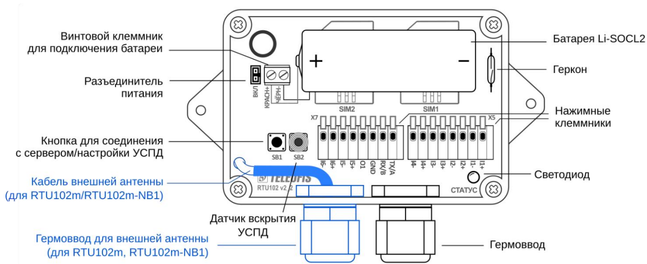
Рис. 4. УСПД серии RTU102. Размещение компонентов на плате.
