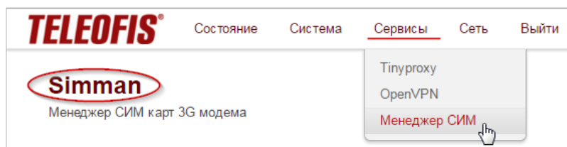
Рис. 42. Менеджер SIM-карт.
